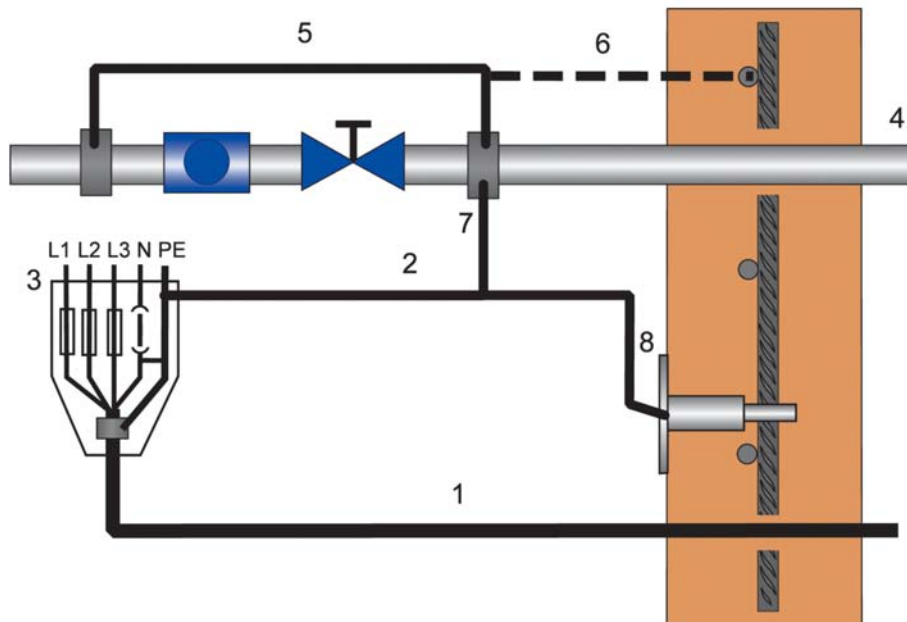
Abb. 4 Anschluss des alternativen Erders 8 und Verschiebung des Anschlusses des Erdungsleiters an die Wasserleitung 7.
